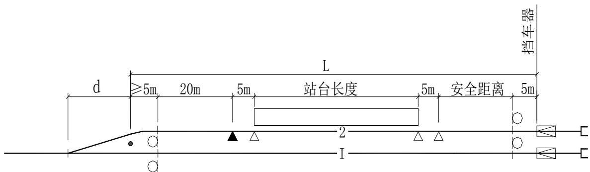
说明图 3.2.7-2 尽头式到发线有效长度示意图
