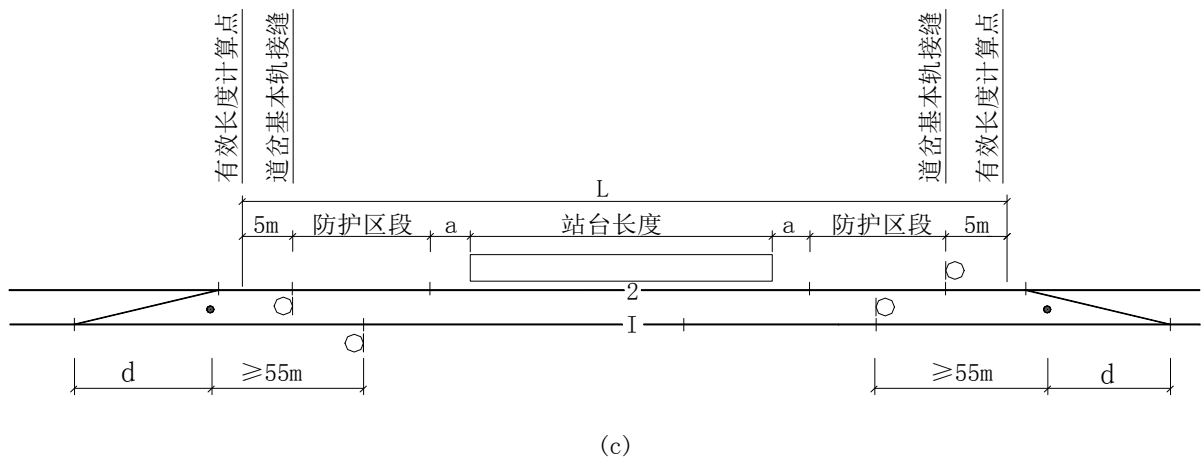
说明图 3.2.5-1 贯通式到发线有效长度示意图 L —到发线有效长度； a —防护区段距站台端的距离； d —岔心至警冲标的距离，按建筑限界计算确定
